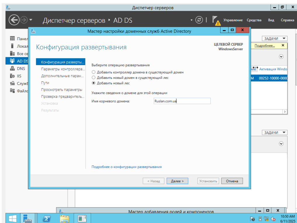
Рис.7 Створення нового лісу
