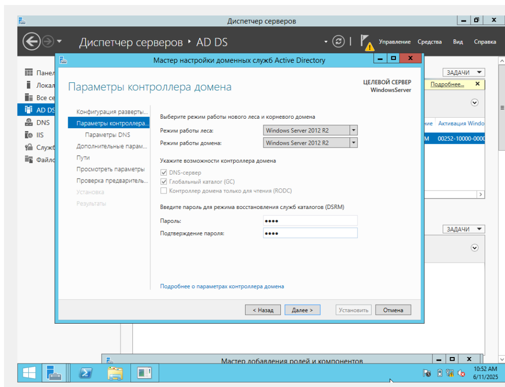
Рис.8 режим зворотної сумісності з попередніми версіями служби AD
